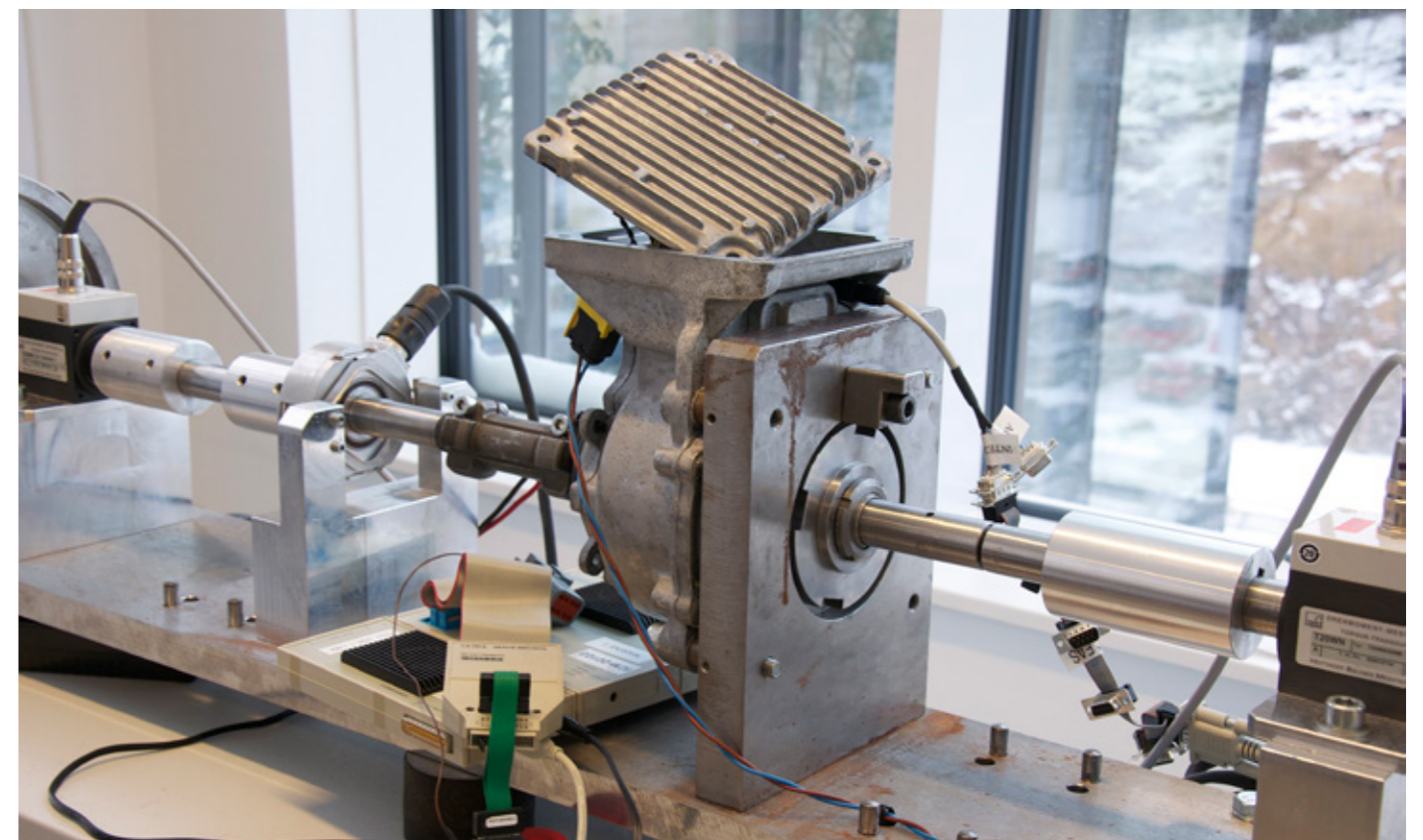
Volvo Dynamic Steering, styrsystemet som Jean-Claude Van Damme marknadsförde ståendes i split mellan två lastbilar. Se Volvo Trucks film på www.youtube.com/watch?v=M7Flvfx5J10
